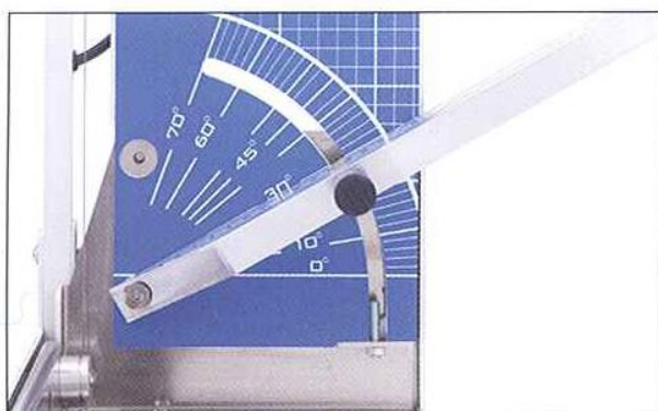
Staffa di conduzione per tagli ad angolo leggera e facile da fissare
